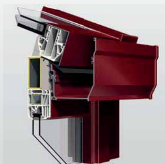
punto di gronda ad elevato isolamento termico ed acustico
