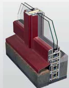
attacchi a pavimento termicamente isolati e resistenti al freddo grazie a profili pluricamera
