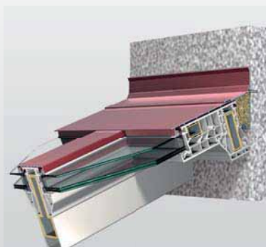
attacchi al tetto innovativi e collaudati
